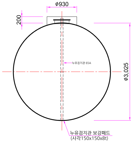
50,000L 탱크 정면도 scale 1:60(A3)
