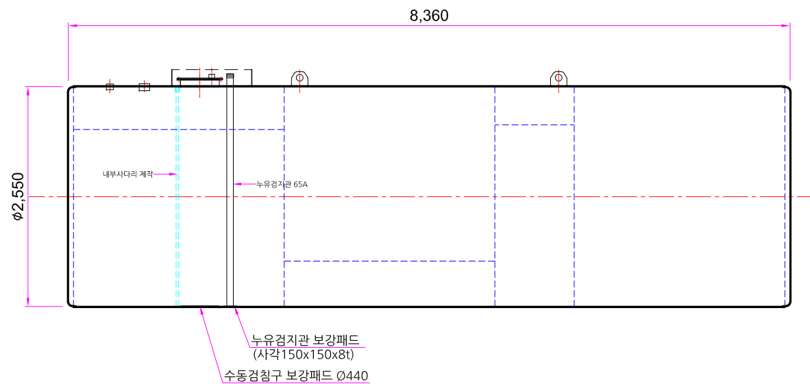
40,000L 탱크 단면도 scale 1:60(A3)
