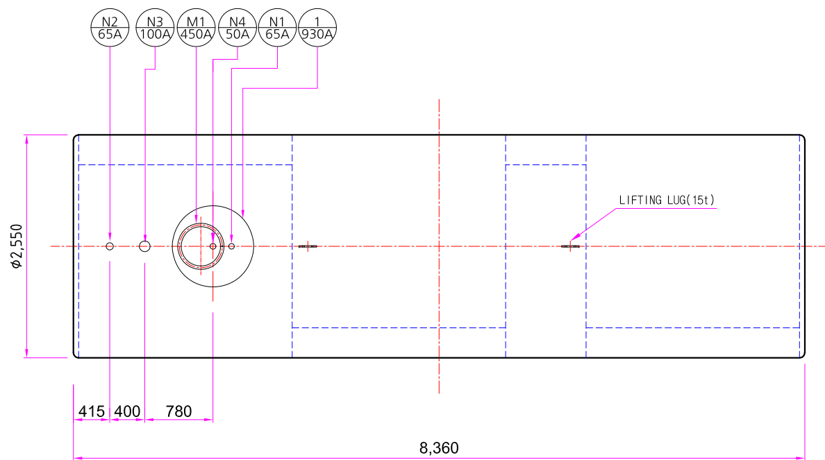
40,000L 탱크 평면도 scale 1:60(A3)
