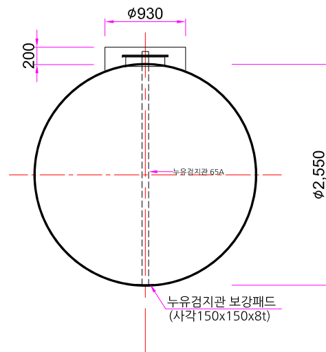
40,000L 탱크 정면도 scale 1:60(A3)
