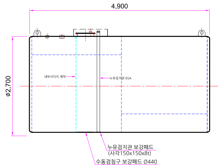
24,000L 탱크 단면도 scale 1:60(A3)
